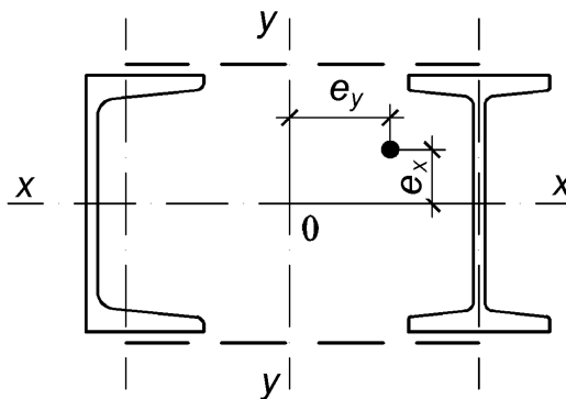
Рисунок 10.1 – Схема наскрізного перерізу стрижня з двома суцільноствінчастими гілками
