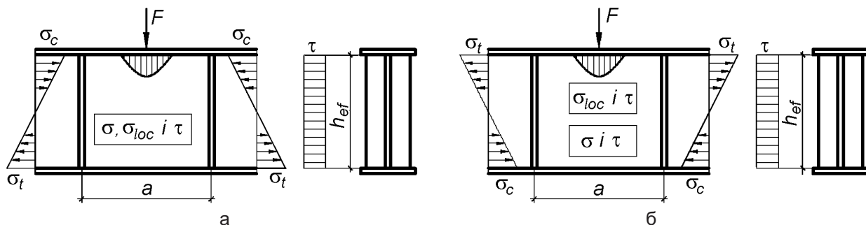
а – при прикладенні зосередженого навантаження до стиснутого пояса; б – те саме до розтягнутого
