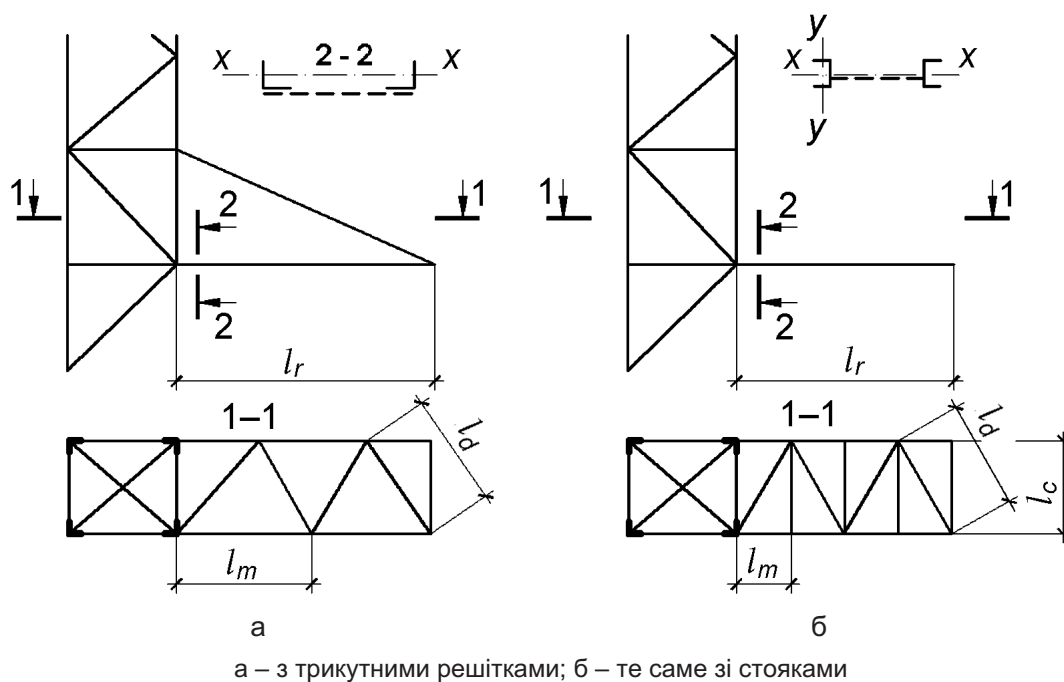
Рисунок 19.1 – Схеми траверс
