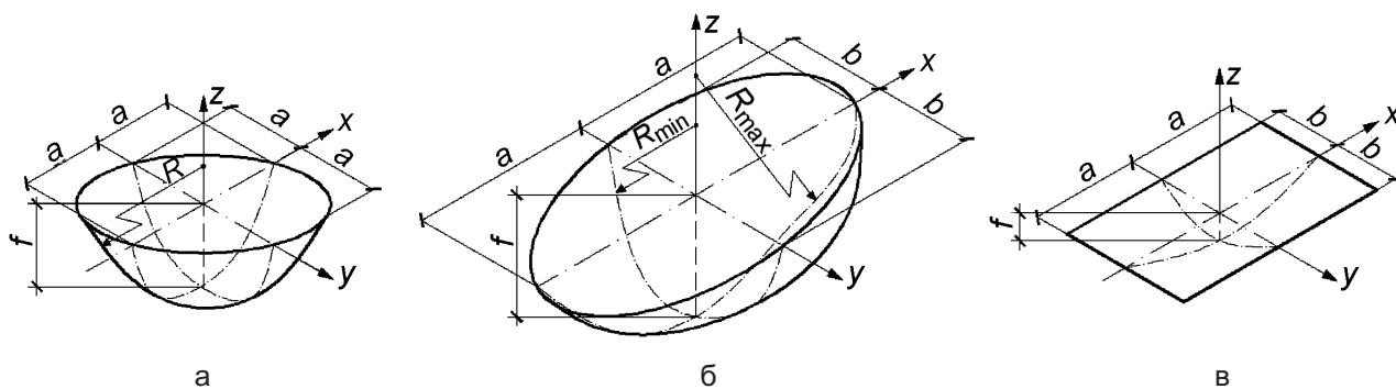
Рисунок 14.4 – Геометрія поверхні оболонки позитивної гауссової кривизни
