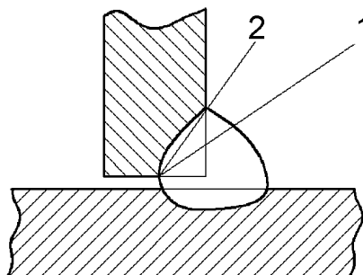
Рисунок 16.4 – Поперечний розріз кутового шва із зазначенням умовних площин руйнування
