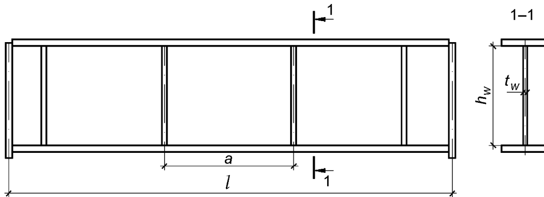
Рисунок 22.1 – Схема балки з гнучкою стінкою
