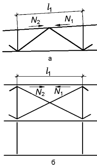
а – схема ферми; б – схема поперечних горизонтальних в'язей між фермами (вид зверху)
