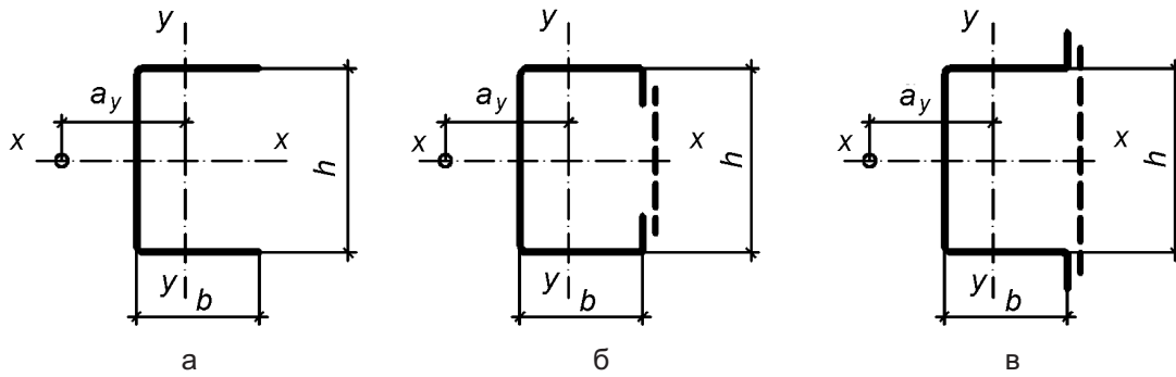
Рисунок 8.1 – Схеми перерізів стрижнів
