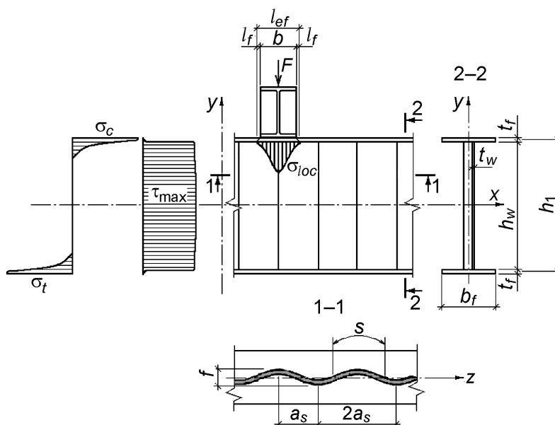
Рисунок 24.1 – Схема елемента з хвилястою (синусоїдною) поперечно-гофрованою стінкою
