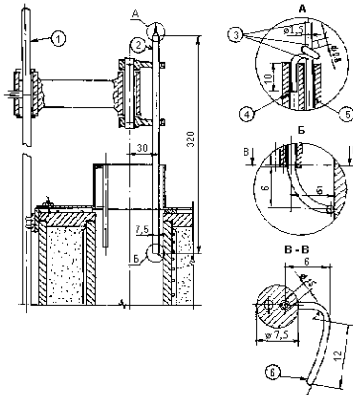
Рисунок А-7 Сканирующий прибор термопары Сканирующее устройство термопары
