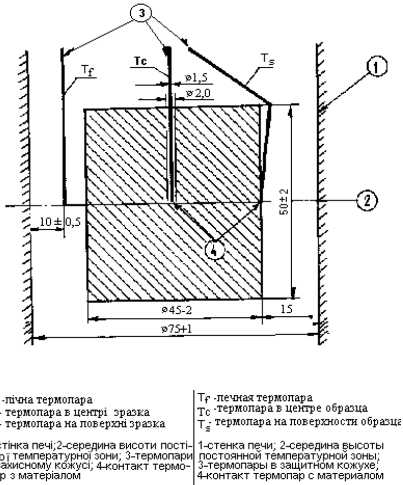
Рисунок А-5 Взаемне розташування печі, зразка і термопар Взаимное расположение печи, образца и термопар
